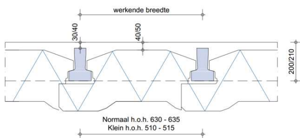
Doorsnede
