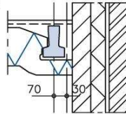
DETAIL - RANDLIGGER
