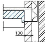
DETAIL - EINDOPLEGGING ZONDER RANDKIST
