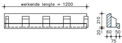
PS-randbekisting RA
