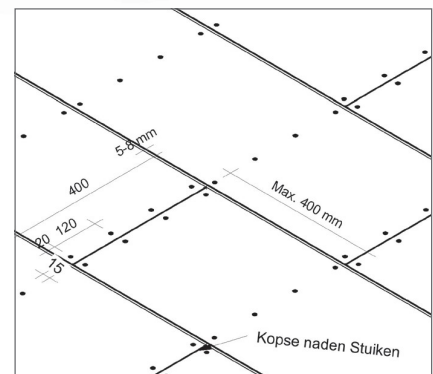
Stucplaten 400 mm breed 4 schroeven per regel
