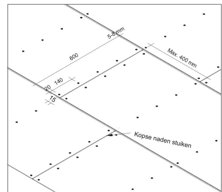
Stucplaten 600 mm breed 5 schroeven per regel
